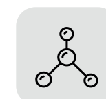
Elettrostatica
